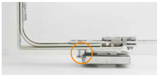
Ergot à épaulement réglable en hauteur et gâche de sécurité
