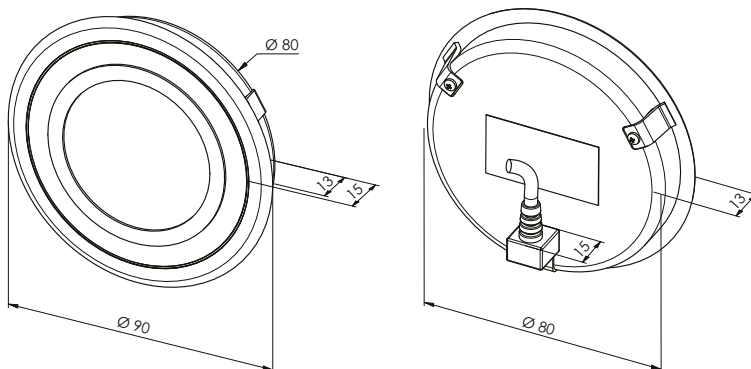
Ausschnitt Einbau Aufsatzmontage: Découpe montage rapporté:
