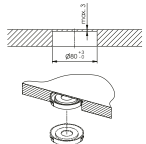
Ausschnitt unsichtbarer Einbau (unterhalb der Arbeitsplatte): Découpe montage invisible (sous le plan de travail):
