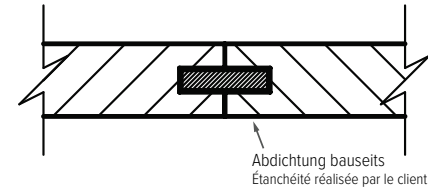
Detail Z / Détail Z
