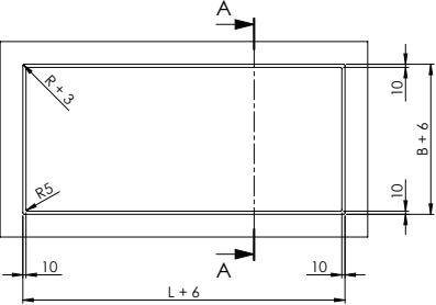
Formbeispiel / Exemple de forme
