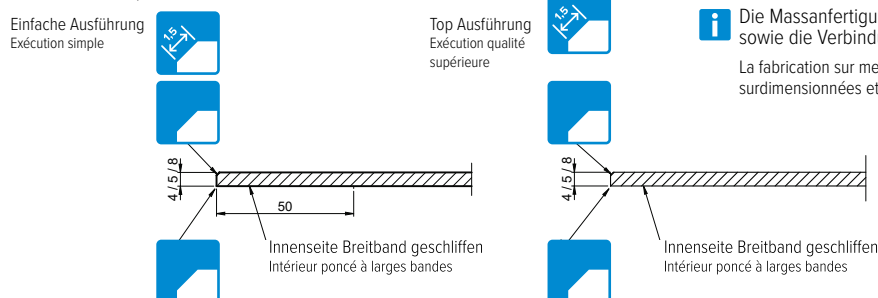
Schnitt A-A / Coupe A-A
