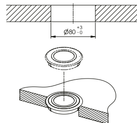
Ausschnitt Einbau Aufsatzmontage: Découpe montage rapporté:
